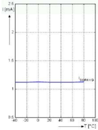
V_S=2.7V 时, I_{SOPAVG} \sim T_A 曲线
