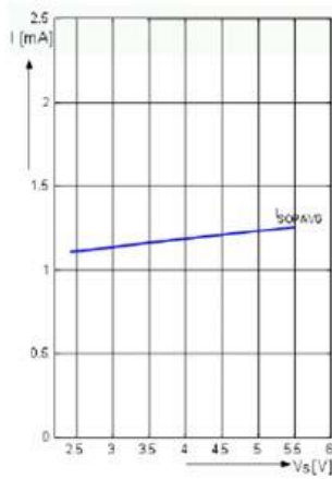
T_A=20^{\circ}C 时, I_{SOPAVG} \sim V_S 曲线
