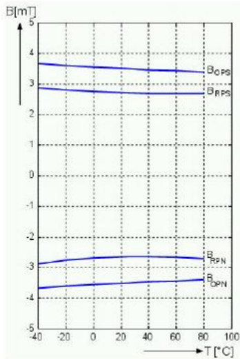
V_S=2.7V 时, B \sim T_A 曲线
