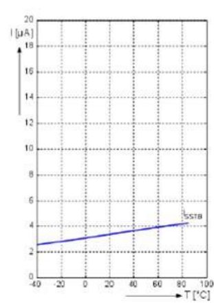
V_S=2.7V 时, I_{SSTB} \sim T_A 曲线
