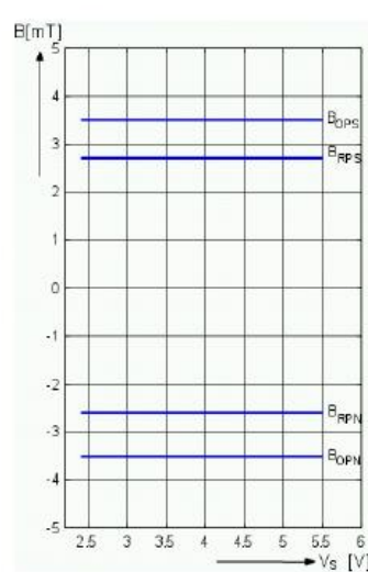
T_A=20^{\circ}C 时, B \sim V_S 曲线
