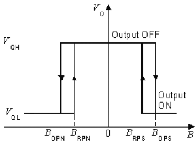
输出开关特性曲线
